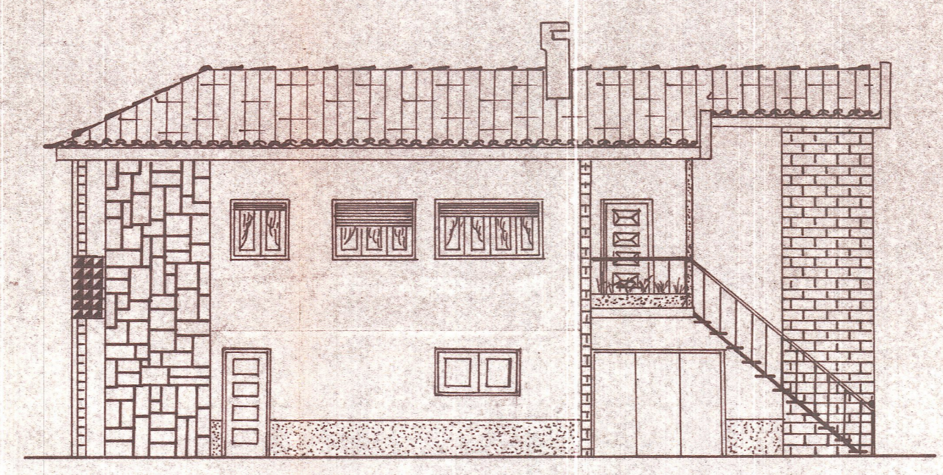
ALÇADO PRINCIPAL
