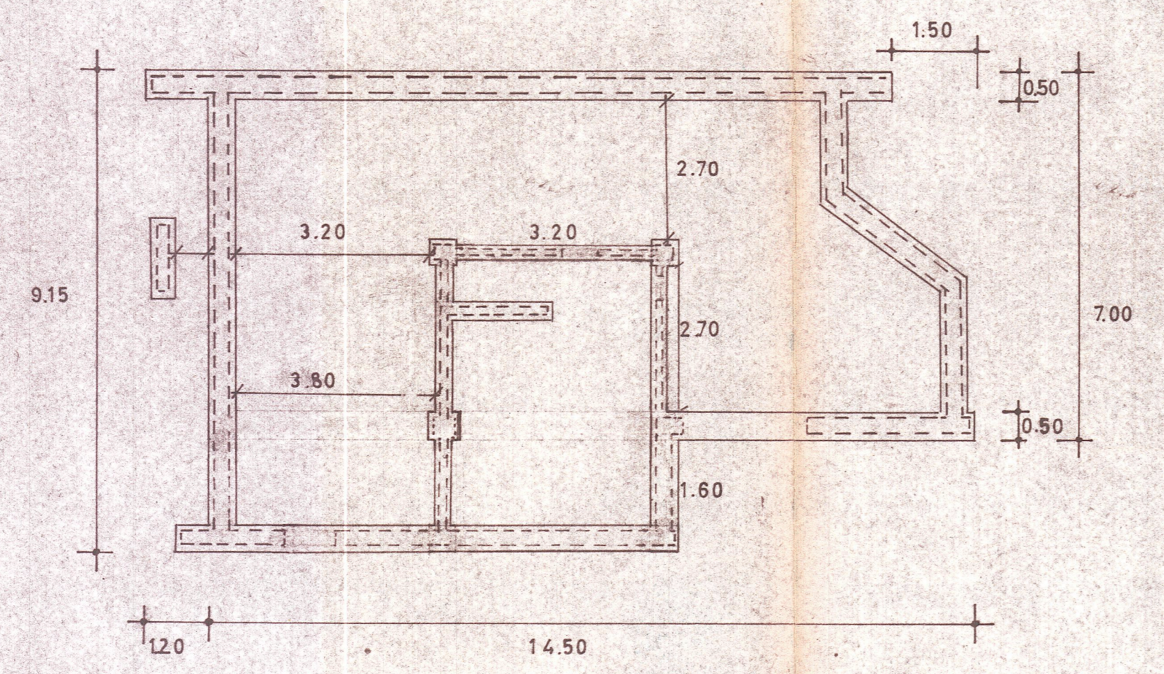
PLANTA DAS FUNDAÇÕES
