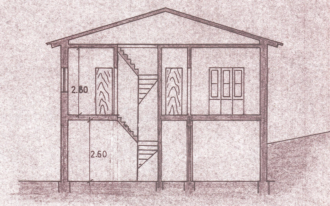
CORTE A-B
