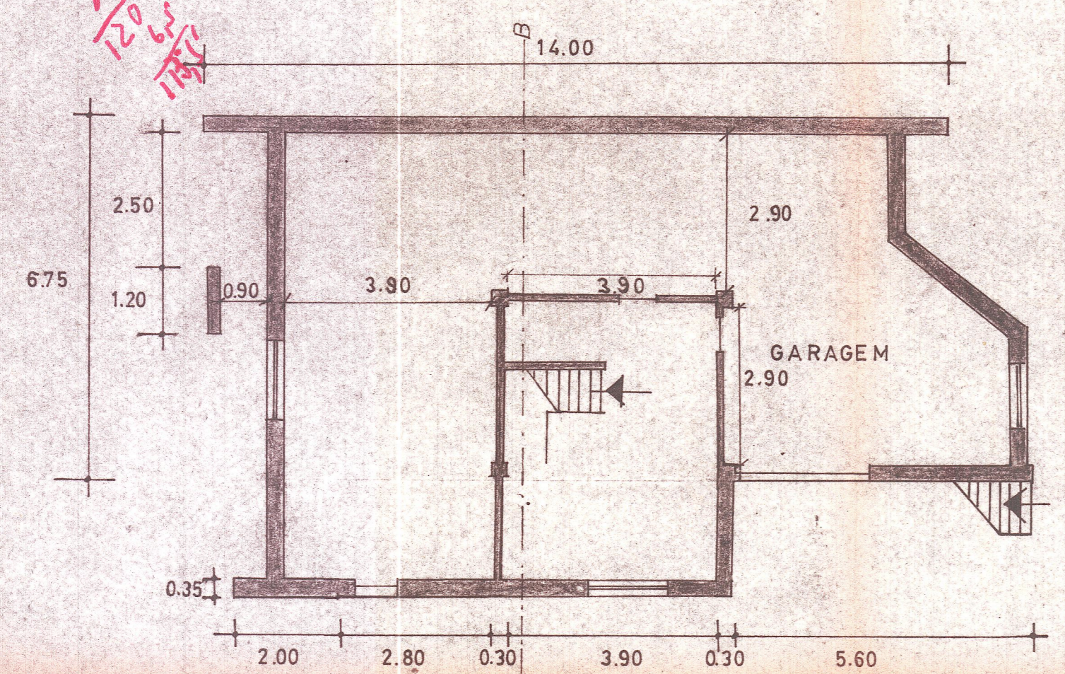
PLANTA DO 1º PISO
