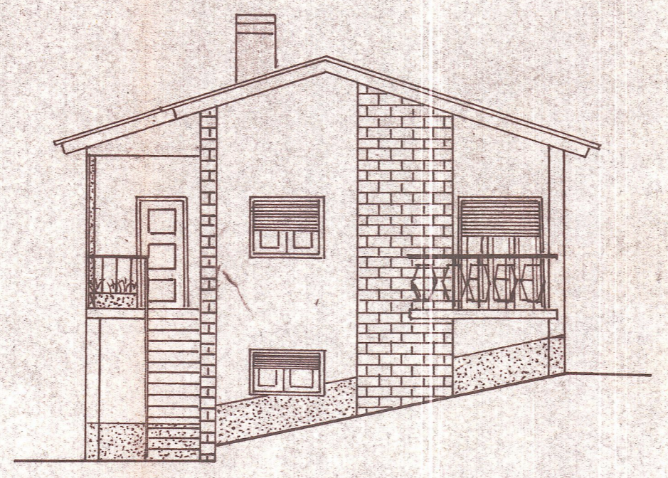
ALÇADO LATERAL DIREITO
